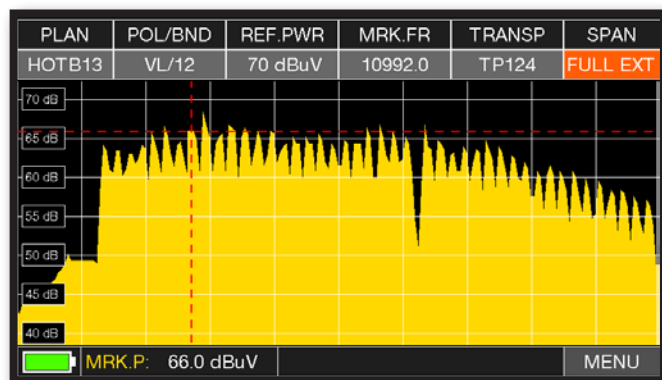
Spettro SAT SPAN "Full EXT" (da 700 a 2700 MHz).
