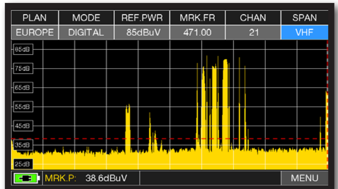
SPETTRO CATV SPAN VHF.
