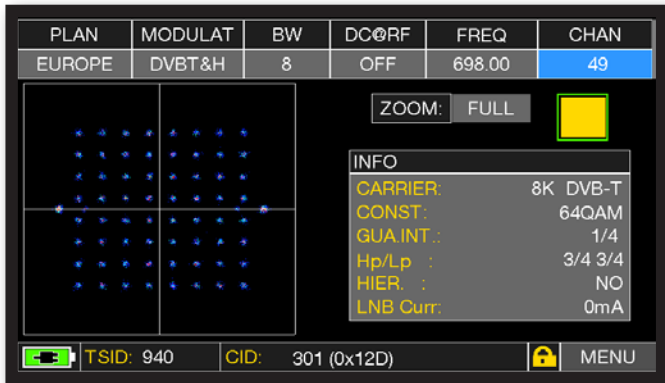
Costellazione DVB-T
