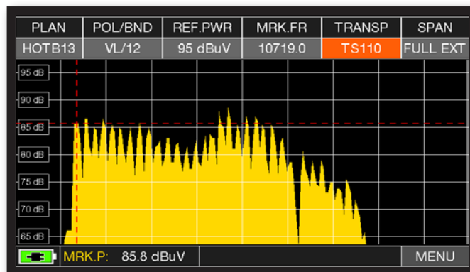
Spettro "SAT" SPAN FULL EXT (da 700 a 2700 MHz) con LNB universale.
