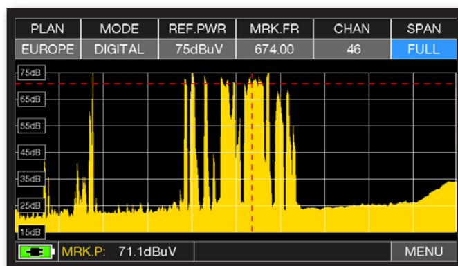
Spettro "TV" SPAN FULL (da 30 a 1.000 MHz).
