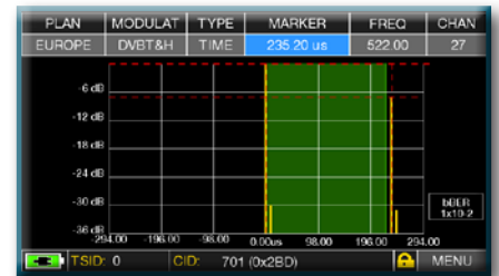
Fig. 3: RICEZIONE MARGINALE (o IMPOSSIBILE): * 2 ECHI presenti all'esterno della maschera dell' Intervallo di Guardia, provenienti da una distanza di: 1° eco: 70,56 Km, pari ad un ritardo di 232,20 \mu s .
